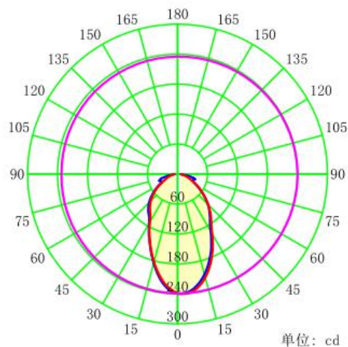
配光曲线
